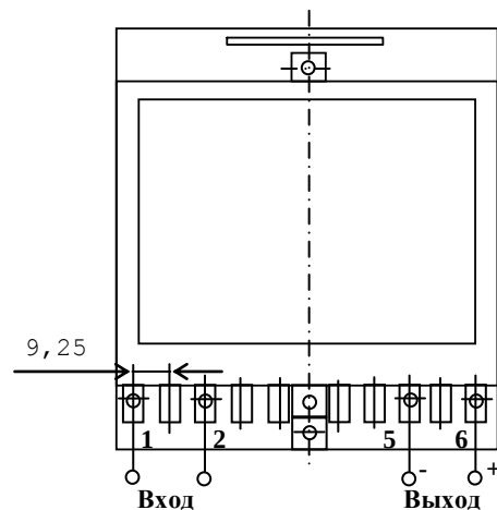
Рисунок А.1 – габаритные и установочные размеры ИП
