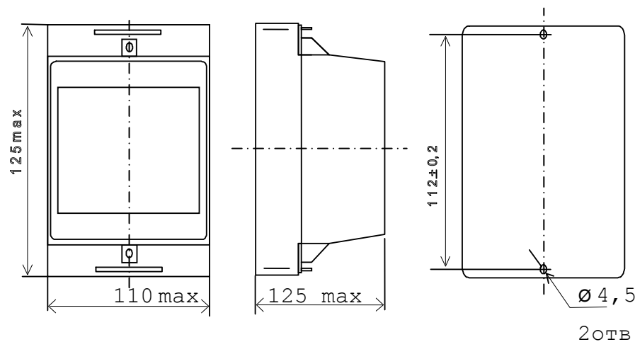
Рисунок А.1 – габаритные и установочные размеры ИП
